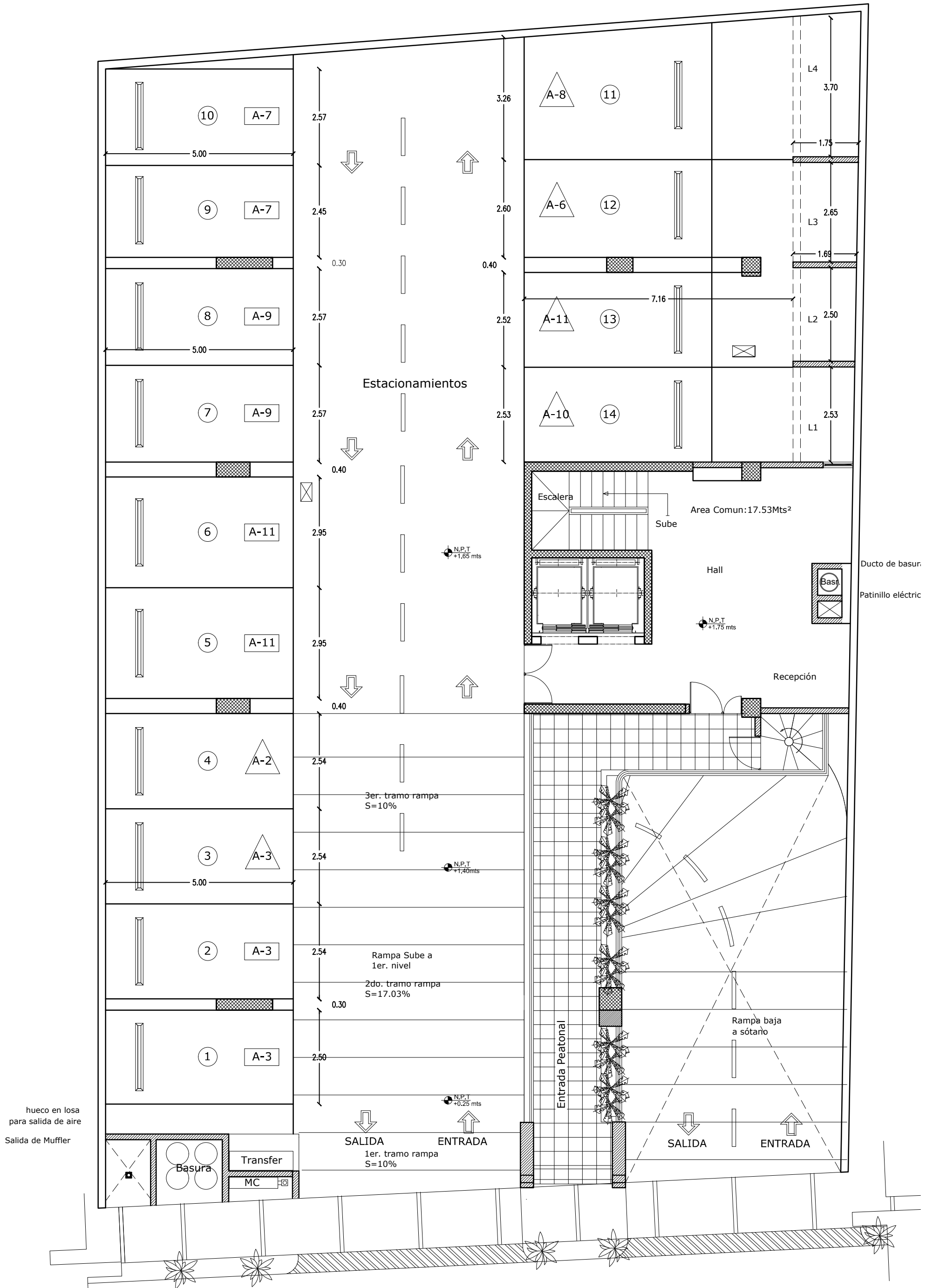
P2 PLANO ARQUITECTONICO D "1er. Nivel" Escala: 1 : 75
